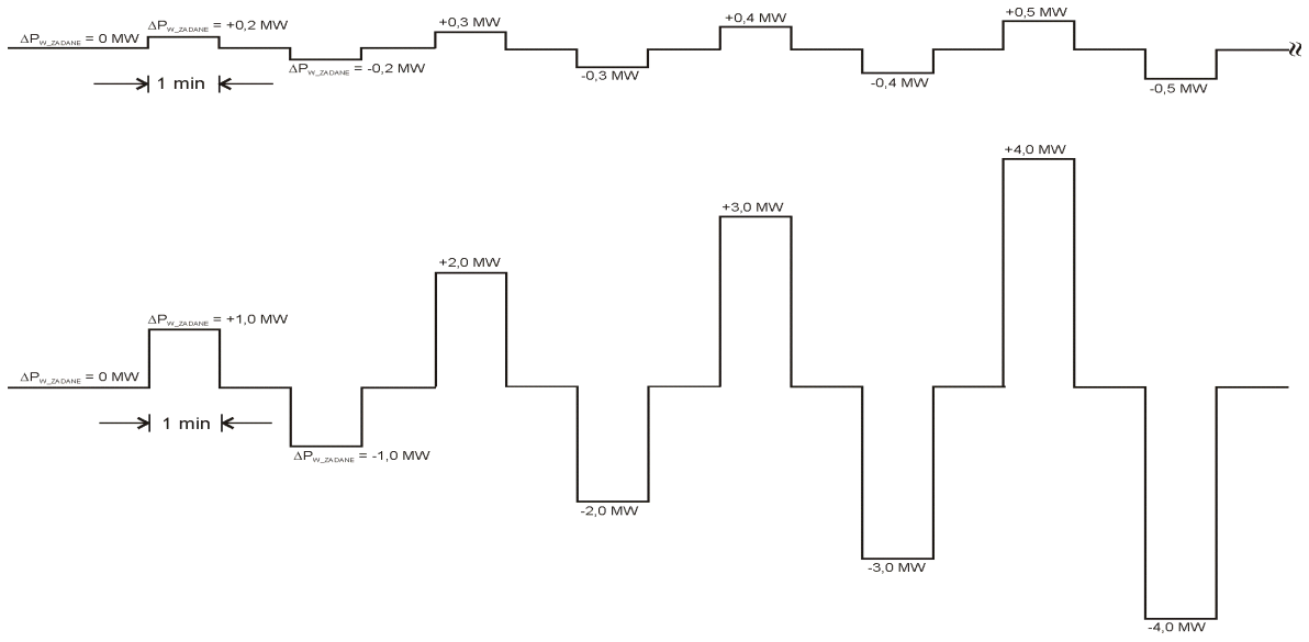
Rys. 1 sprawdzenie rozdzielczości regulacji odbudowy częstotliwości.
