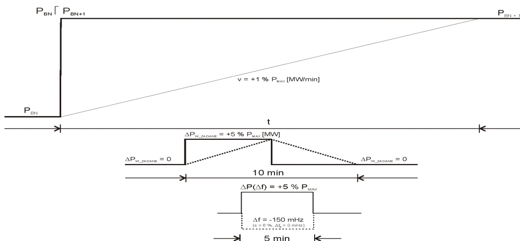
Rys. 9 Sprawdzenie odpowiedzi współdziałania regulacji odbudowy częstotliwości oraz regulacji FSM na tle zmieniającej się mocy bazowej
