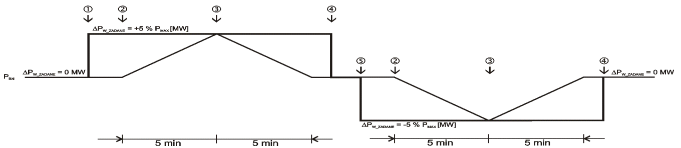
Rys. 2 sprawdzenie działania regulacji wtórnej w odpowiedzi na wymuszenie w torze regulacji wtórnej w trakcie wyłączania i załączania stanu regulacji wtórnej
