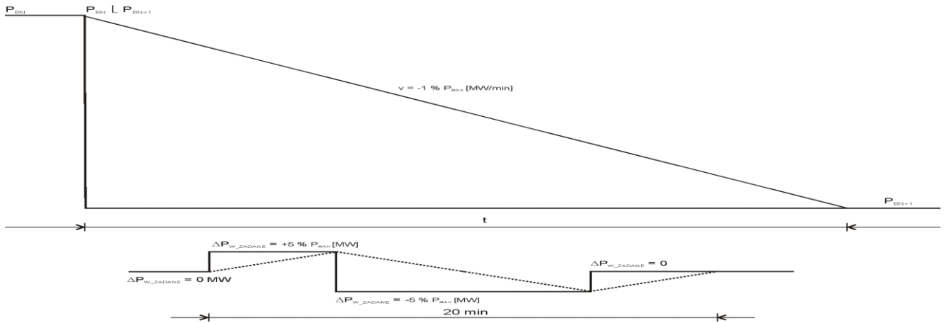
Rys. 10 Sprawdzenie odpowiedzi współdziałania regulacji odbudowy częstotliwości na tle zmieniającej się mocy bazowej
