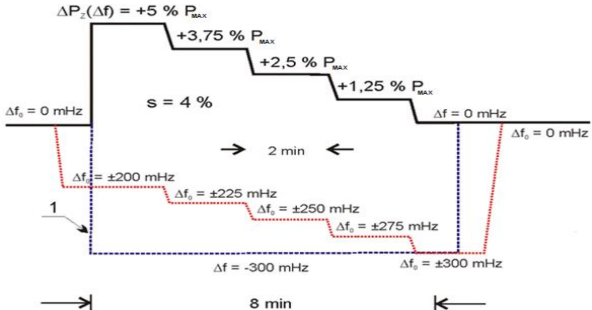
Rys. 4 Sprawdzenie odpowiedzi częstotliwościowej przy zmianach: strefy nieczułości odpowiedzi częstotliwościowej, statyzmu oraz odchyłki częstotliwości
