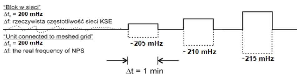
Rys. 1 Sprawdzenie niewrażliwości odpowiedzi częstotliwościowej.
