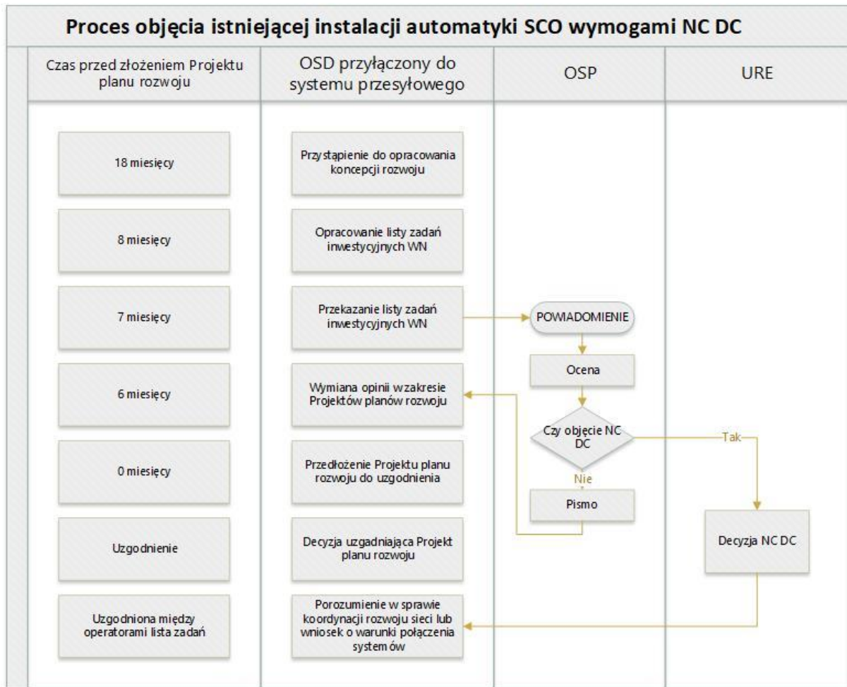
Rys. 1 – Proces objęcia istniejącej instalacji automatyki SCO wymogami NC DC w przypadku modernizacji lub wymiany urządzeń oraz proces określania warunków przyłączenia i zmiany lub zawierania nowej umowy przyłączeniowej
